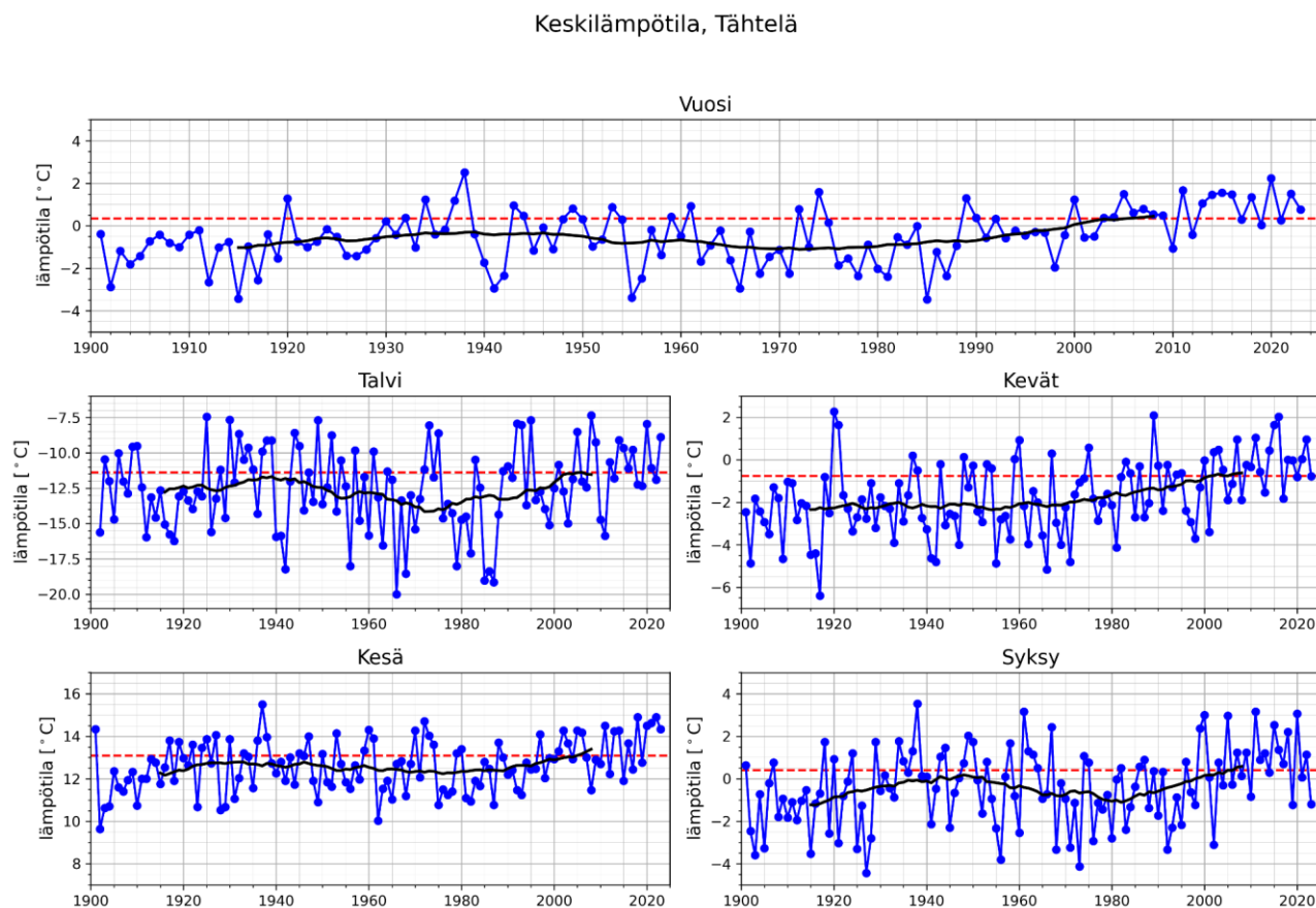
Kuva 11 Keskilämpötila 1901–2023 koko vuodelle sekä vuodenajoittain Sodankylän Tähtelän sääasemalla. Siniset pisteet ovat vuosittaisia arvoja, punainen katkoviiva kuvaa ilmastollisen vertailukauden 1991–2020 keskiarvoa ja musta viiva on 30-vuoden liukuva keskiarvo.
