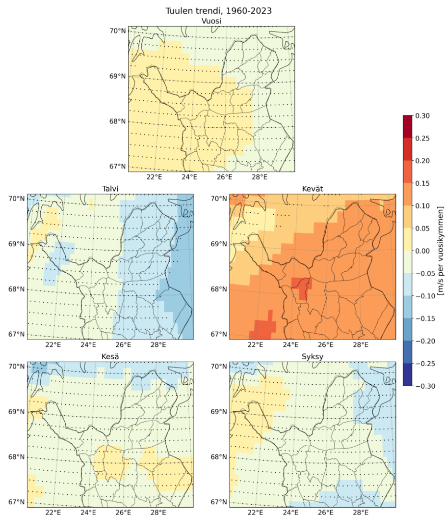
Kuva 18 925-hPa painepinnan tuulen nopeuden trendi jaksolla 1960–2023 koko vuodelle sekä vuodenaikojen
