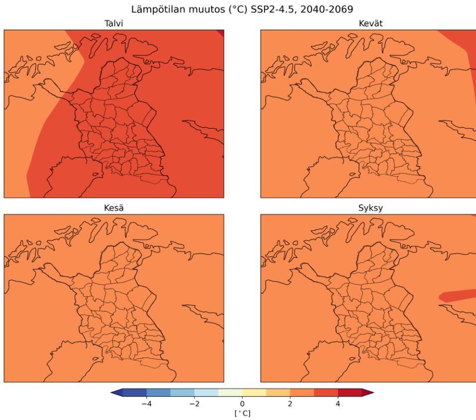
Kuva 26 Lämpötilan muutos (Celsius-asteina) vuodenajoinnain jaksolle 2040–2069 verrattuna jaksoon 1981–2010 keskinkertai- sen päästöskenaarion (SSP2-4.5) pohjalta
