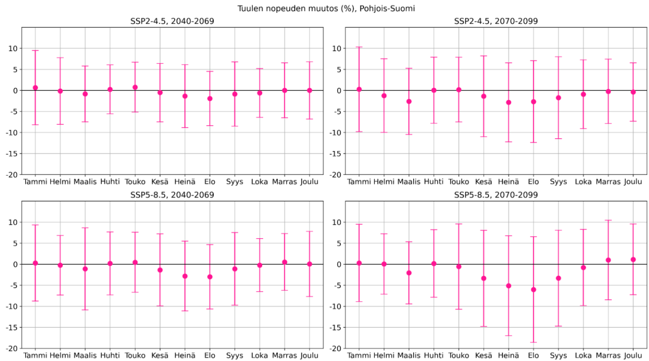
Kuva 34 Tuulen nopeuden muutos (prosentteina) kuukausittain jaksoille 2040–2069 ja 2070–2099 verrattuna jaksoon 1981–2010 keskinkertaisen päästöskenaarion (SSP2-4.5) ja voimakkaan päästöskenaarion (SSP5-8.5) pohjalta
