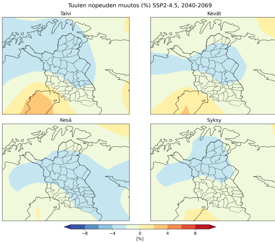
Kuva 32 Tuulen nopeuden muutos (prosentteina) vuodenajoinnain jaksolle 2040–2069 verrattuna jaksoon 1981–2010 keskinkertaisen päästöskenaaron (SSP2-4.5) pohjalta
