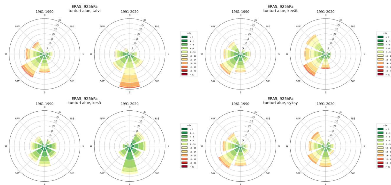
Kuva 25 Ilmastollisten vertailujaksojen 1961–1990 ja 1991–2020 925-hPa painepinnan tuuliruusut vuodenajoittain tunturialueella
