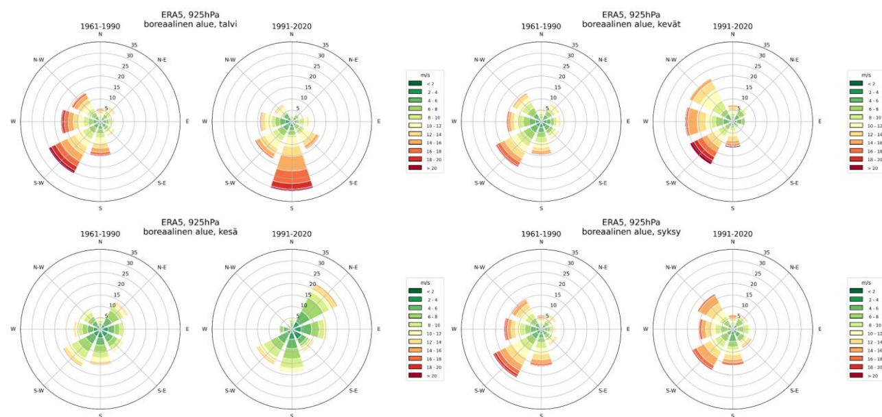
Kuva 23 Ilmastollisten vertailujaksojen 1961–1990 ja 1991–2020 925-hPa painepinnan tuuliruusuut vuodenajoittain boreaalisella alueella
