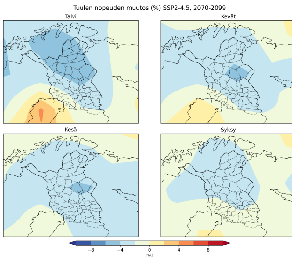
Kuva 33 Tuulen nopeuden muutos (prosentteina) vuodenajoittain jaksolle 2070–2099 verrattuna jaksoon 1981–2010 keskinkertaisen päästöskenaarion (SSP2-4.5) pohjalta
