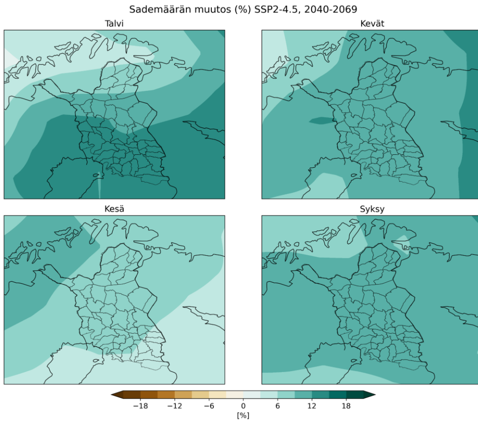
Kuva 29 Sademäärän muutos (prosentteina) vuodenajoittain jaksolle 2040–2069 verrattuna jaksoon 1981–2010 keskinäisen päästöskenaarion (SSP2-4.5) pohjalta
