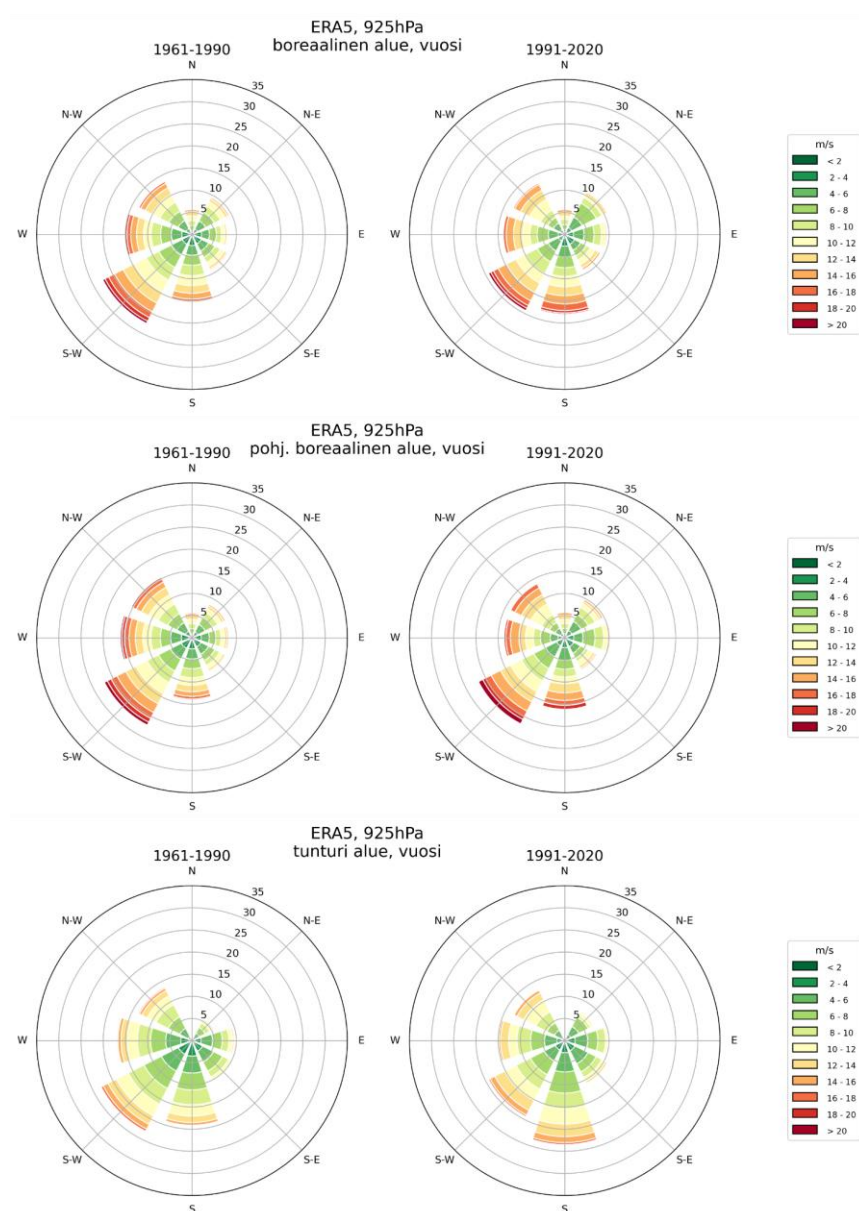
Kuva 22 Ilmastollisten vertailujaksojen 1961–1990 ja 1991–2020 925-hPa painepinnan tuuliruusut koko vuodelle
