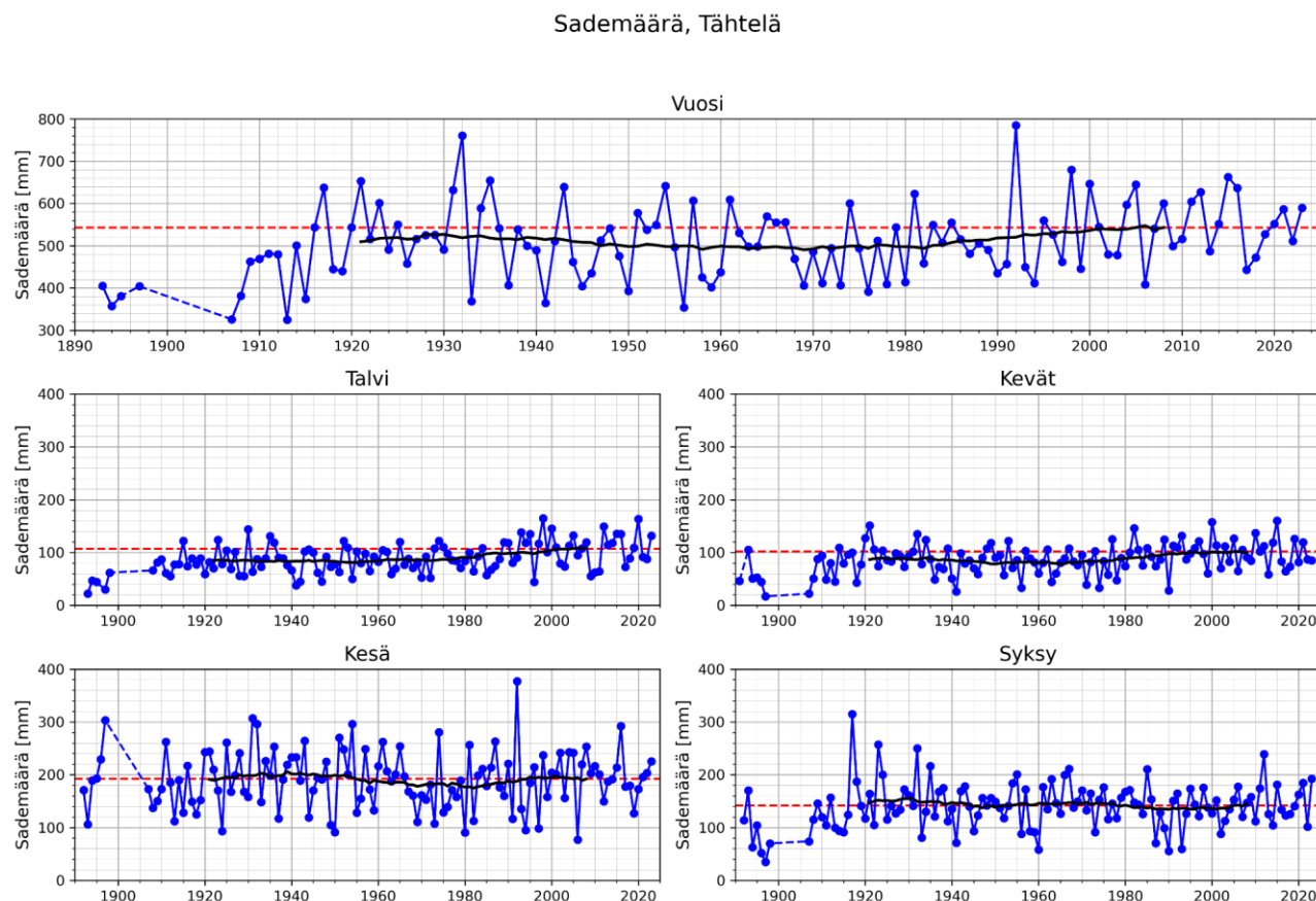
Kuva 17 Sademäärä 1893–2023 koko vuodelle sekä vuodenajoittain Sodankylän Tähtelän sääasemalla. Siniset pisteet ovat vuosittaisia arvoja, punainen katkoviiva kuvaa ilmastollisen vertailukauden 1991–2020 keskiarvoa ja musta viiva on 30-vuoden liuku keskiarvo.
